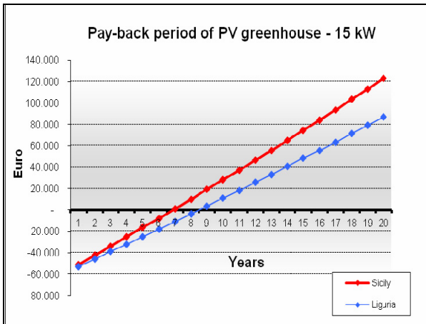
Fig.1 - Comparison of pay-back period for PV greenhouses located in different climatic areas of Italy in Italy (Source: Report “Stato dell’arte e prospettive di sviluppo delle tecnologie per la produzione di Energia Elettrica, di Calore e di Biocarburanti e delle tecnologie per l’Efficienza Energetica”. ENEA, January 2012 (in Italian).
